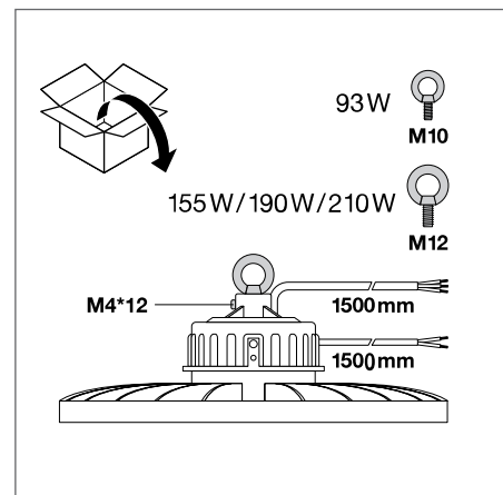
Версии DALI
